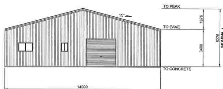
4 ENDWALL EXTERIOR ELEVATION 6 SCALE: 1 = 200
