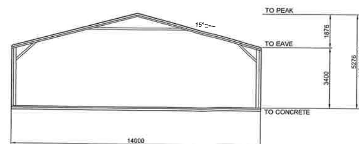
3 ENDWALL EXTERIOR ELEVATION 6 SCALE: 1 = 200
