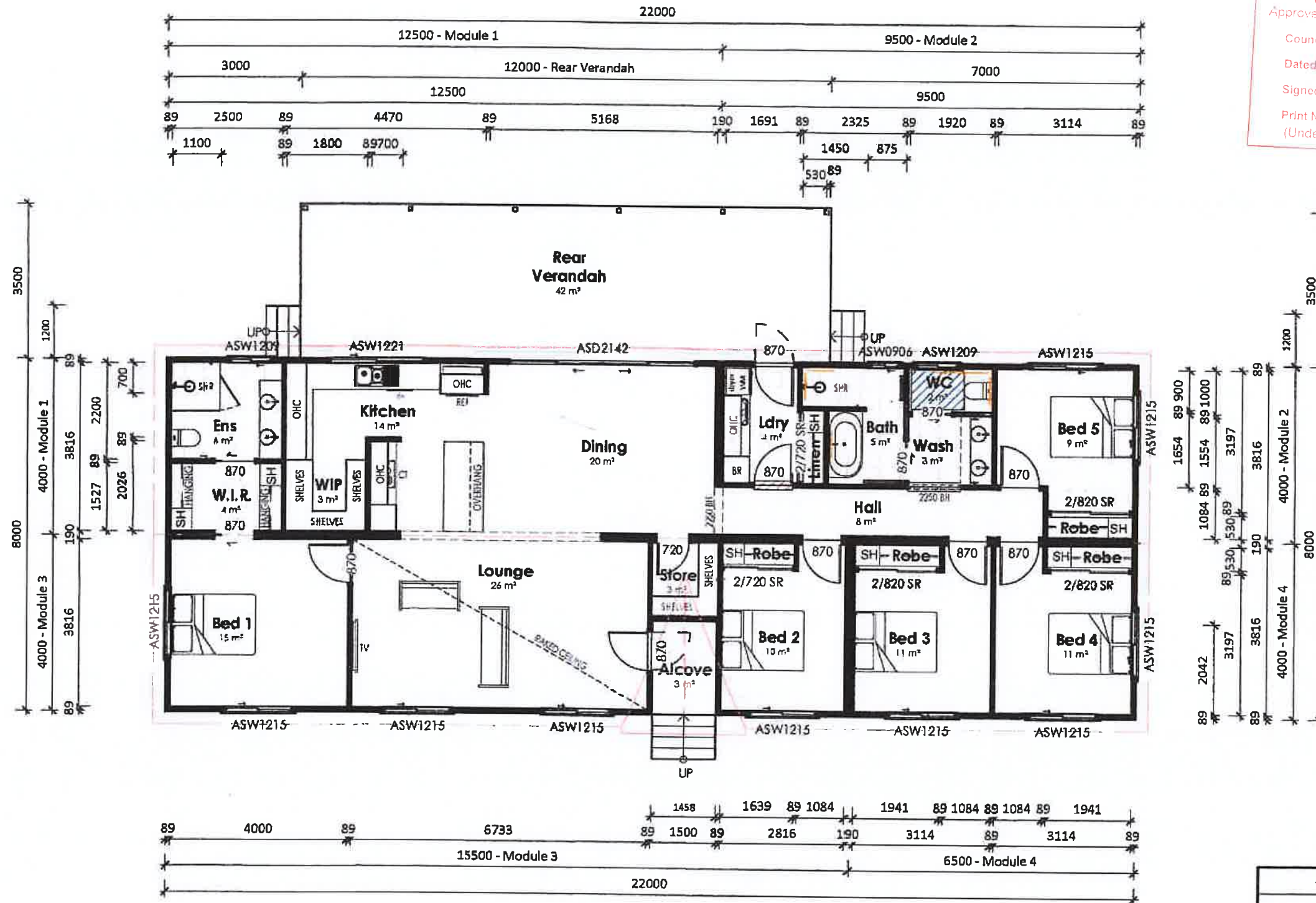
Plan Floor Plan 1 : 100
